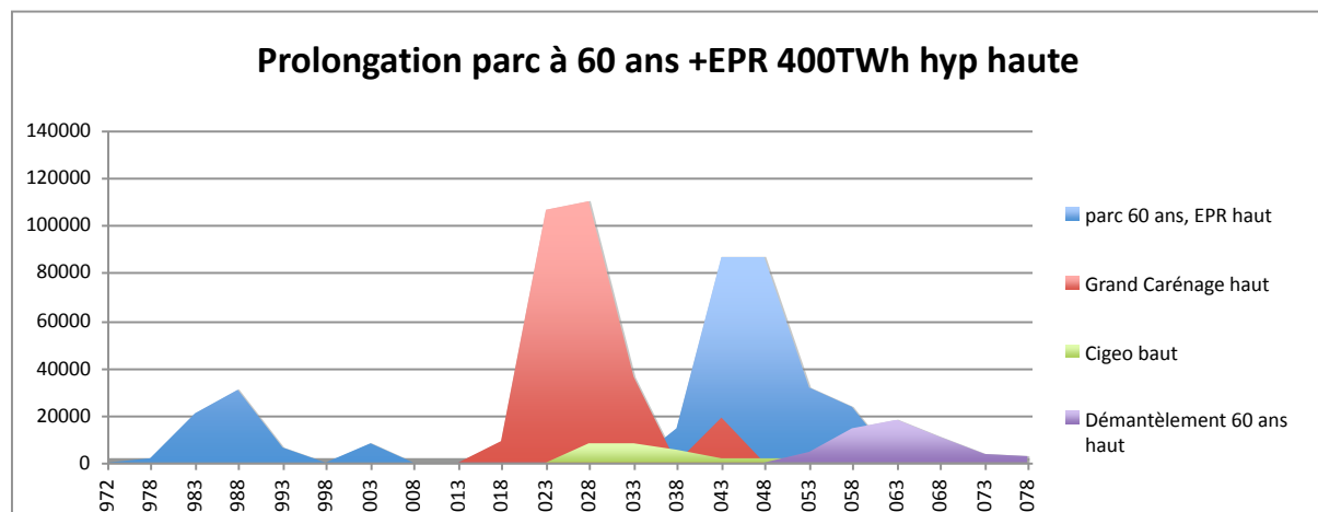
Figure 6 : parc prolongé à 60 ans et renouvelé à partir de 2038 à 400 TWh, EPR haut, carénage haut, Cigeo haut (en M€)
