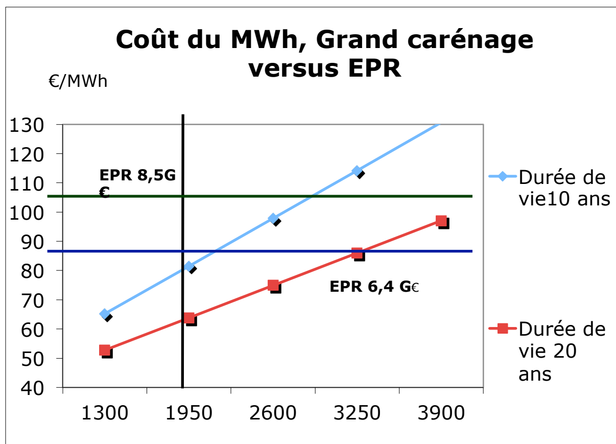
Figure 15 : Coût du MWh EPR et du parc rénové en fonction de celui du grand carénage et de la durée de vie
