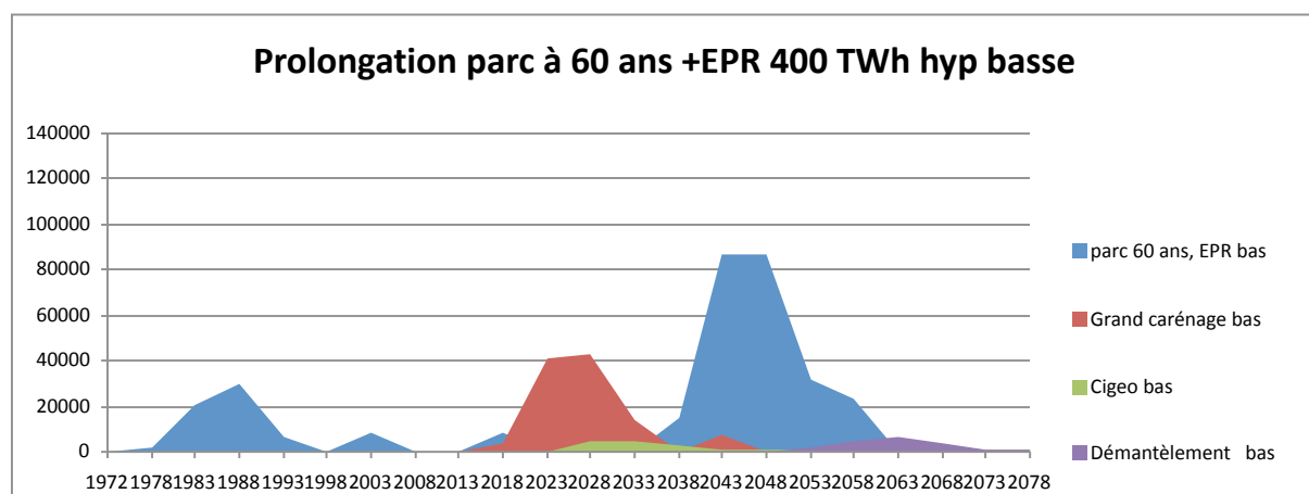
Figure 7 : parc prolongé à 60 ans et renouvelé à partir de 2038 à 400 TWh, EPR bas, carénage bas, Cigeo bas (en M€)
