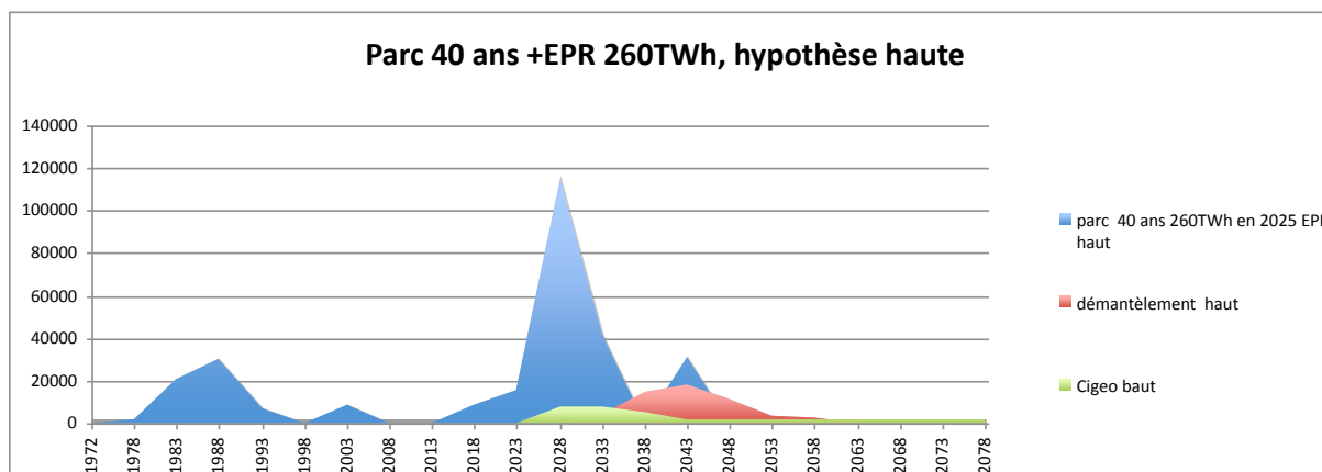
Figure 9 : Chronologie des investissements d'un parc arrêté à 40 ans, renouvelé au niveau de 260 TWh à partir de 2025, EPR haut, démantèlement haut, Cigeo haut (en M€)
