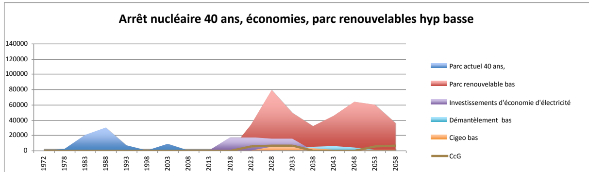
Figure 12 : Chronologie des investissements d'un parc arrêté à 40 ans, avec économies d'électricité et mise en place d'un parc renouvelable et cycles combinés à gaz au niveau de 400 TWh. Hypothèse basse de coût des renouvelables à partir de 2030 (en M€).
