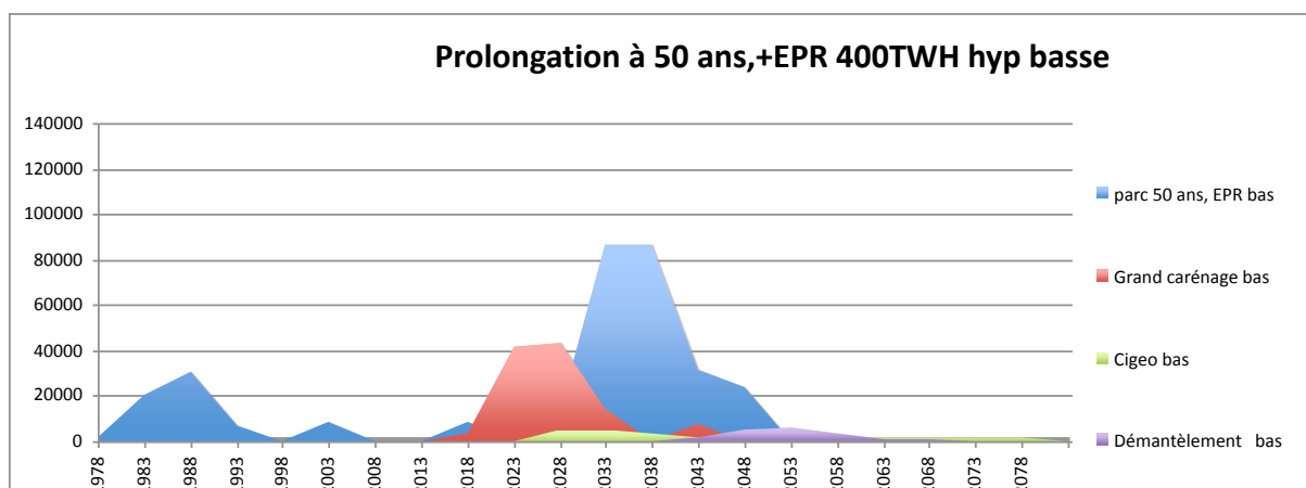
Figure 5 : Parc prolongé à 50 ans, renouvelé à partir de 2028, à 400 TWh, EPR bas, carénage bas, Cigeo bas (en M€)
