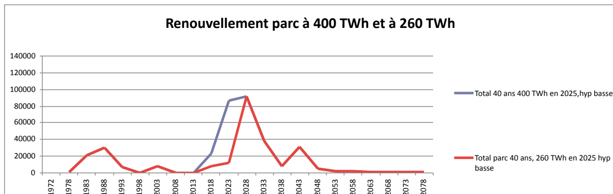
Figure 10 : Chronologies comparées des investissements de deux parcs arrêtés à 40 ans, l'un de 400 TWh, l'autre de 260 TWh, hypothèses basses (en M€)
